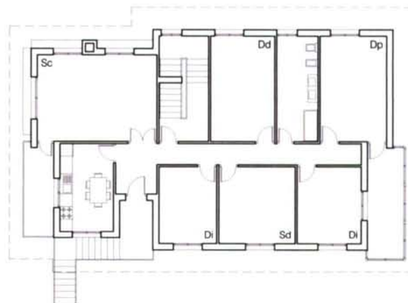
PLANTA PRIMEIRA
