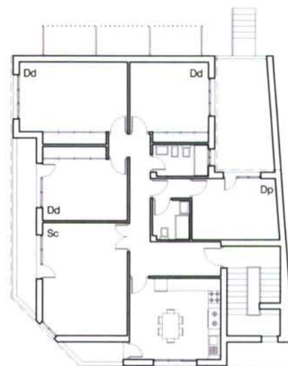
PLANTA PRIMEIRA
