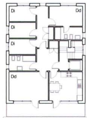
PLANTA PRIMEIRA
