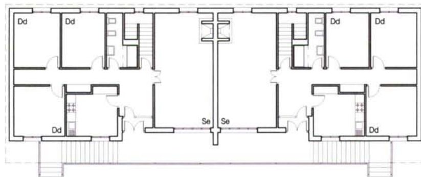
PLANTA PRIMEIRA
