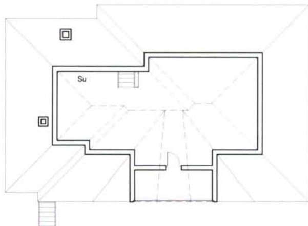
PLANTA BAIXO-CUBERTA
