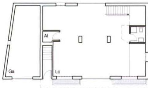
PLANTA BAIXA
