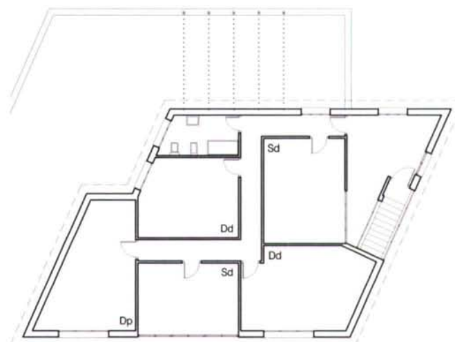
PLANTA PRIMEIRA
