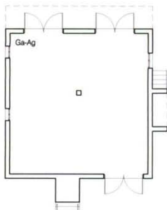
PLANTA SEMISOTO
