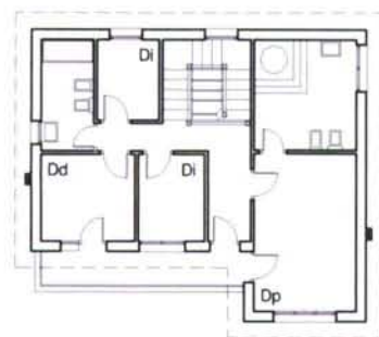
PLANTA PRIMEIRA
