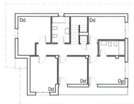
PLANTA SEGUNDA
