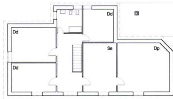
PLANTA PRIMEIRA
