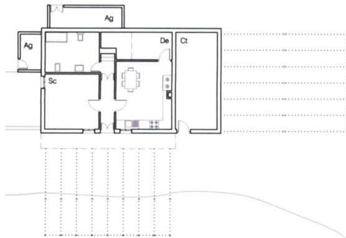
PLANTA BAIXA
