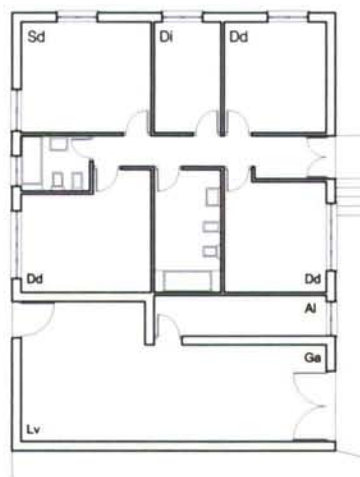
PLANTA SEMISOTO
