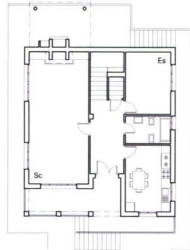
PLANTA BAIXA
