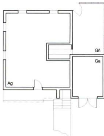
PLANTA BAIXA
