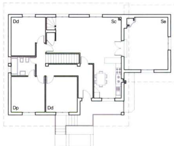
PLANTA BAIXA
