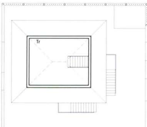
PLANTA BAIXO-CUBERTA
