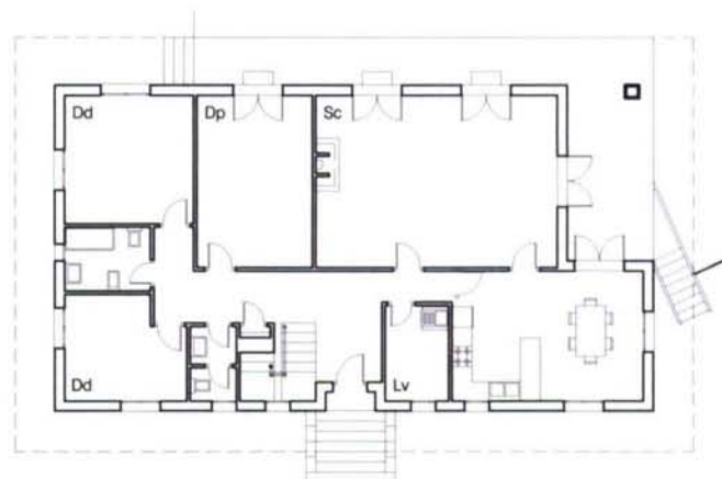
PLANTA BAIXA
