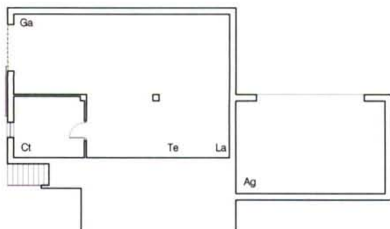
PLANTA SEMISOTO
