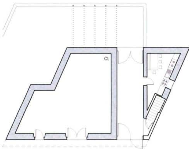
PLANTA BAIXA
