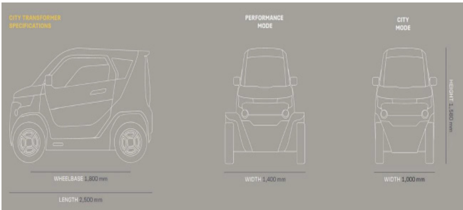
Q Planos del vehículo.
