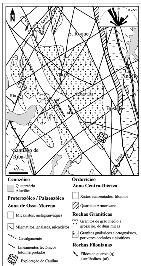
Fig. 7. Enquadramento geológico local da área da exploração de caulino de Bustelo (base geológica reinterpretada de CHAMINÉ, 2000). Diagrama de rosetas: n=51 lineamentos tectónicos.
