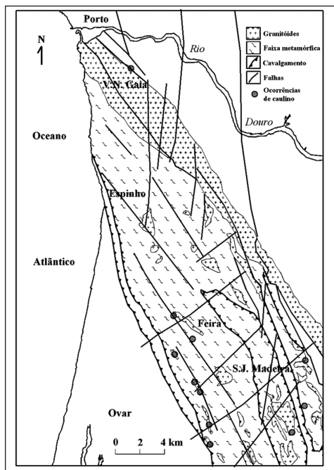
Fig. 8. Esquema de síntese da relação espacial entre os corpos granitoides ao longo de faixas de cisalhamento no caso de estudo (base geológico-estrutural adaptada de CHAMINÉ, 2000).
