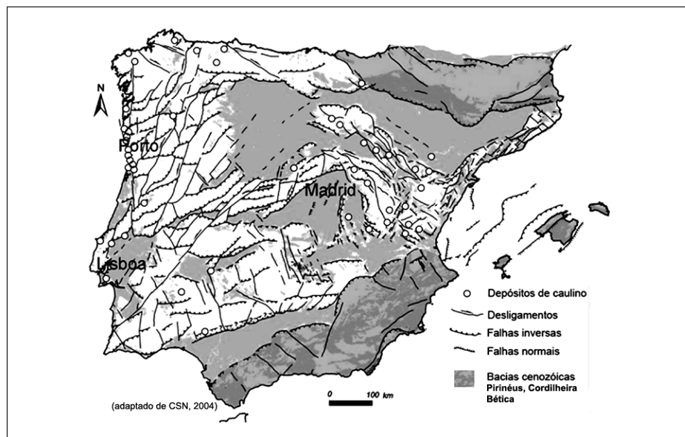
Fig. 1. Ocorrências de caulino na Península Ibérica (adaptado de MME, 1988 e de LOPES VELHO et al., 1998), segundo a base do CSN – Consejo de Seguridad Nuclear, 2004, in De VICENTE et al., 2004).
