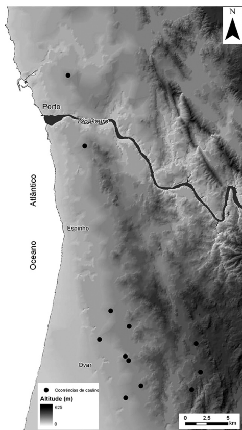
Fig. 3. Modelo Digital de Terreno da área compreendida entre a região do Porto e Ovar, com as principais ocorrências de caulino.
