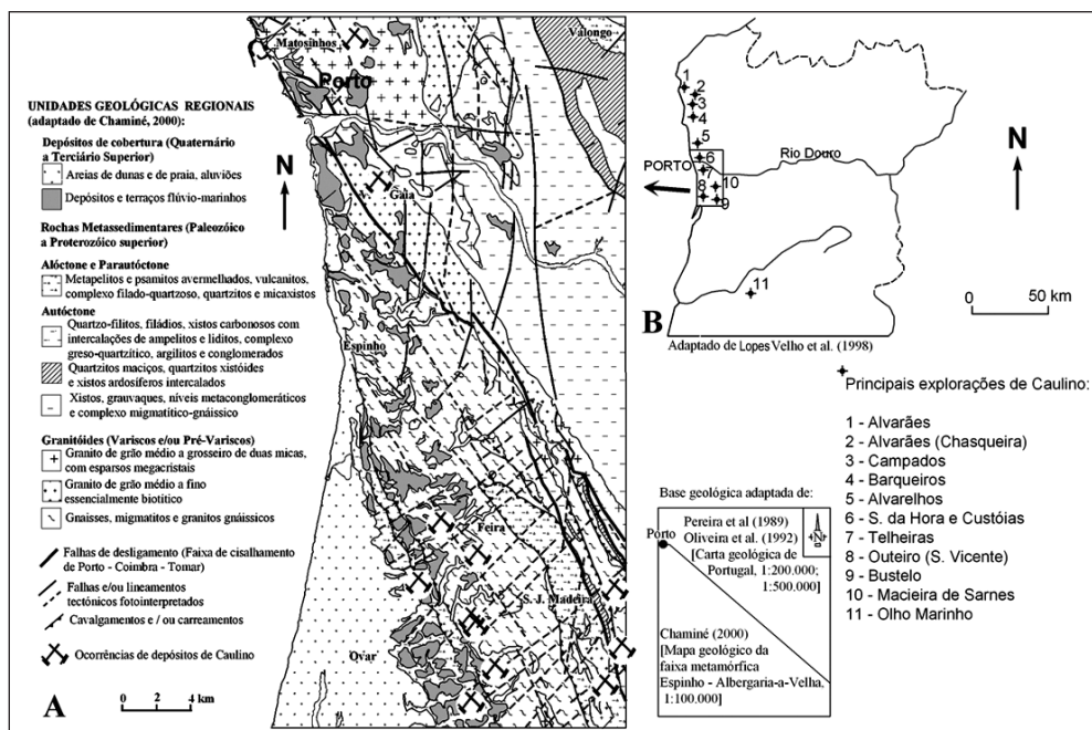
Fig. 2. Enquadramento regional. A) Esboço geológico da faixa metamórfica de Porto-Albergaria-a-Velha, com as ocorrências de caulino (base geológica adaptada de CHAMINÉ, 2000); B) Principais ocorrências de caulino no NW de Portugal (adaptado de LOPES VELHO et al., 1998).
