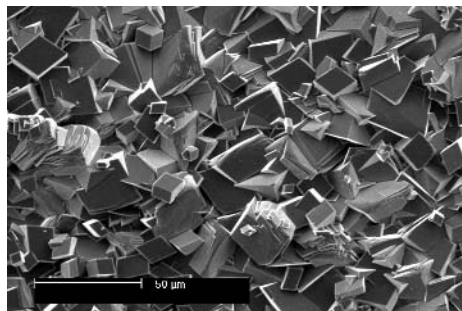
Figura 1. Superficie (110) de un cristal de aragonito recubierta por cristalitas de (Mn,Ca)CO_3 , triangulares.
